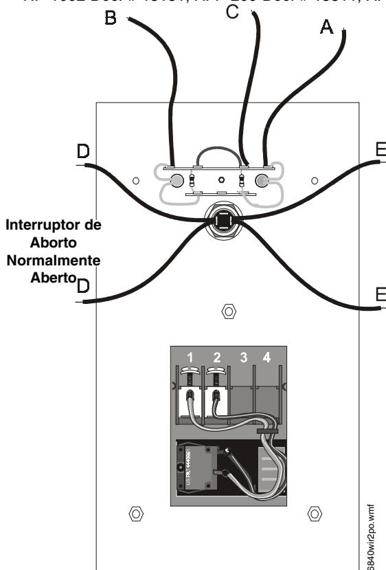
Estação Manual de Descarga de Agente NBG-12LRA (vista traseira)
